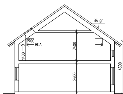
Sektion A-A
