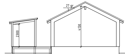
Sektion B-B
