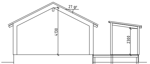
Sektion B-B
