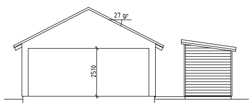
Sektion A-A
