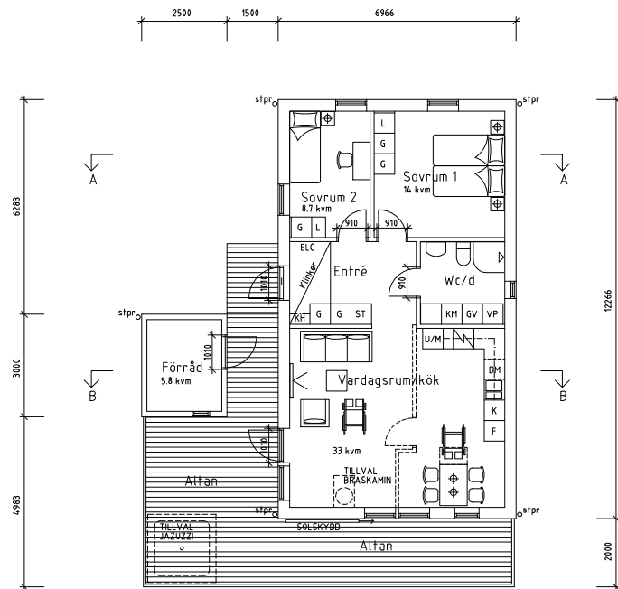
PLAN Mått/utbredning av altan, se märkning. Mått mellan förråd och hus, min 1500 mm.
